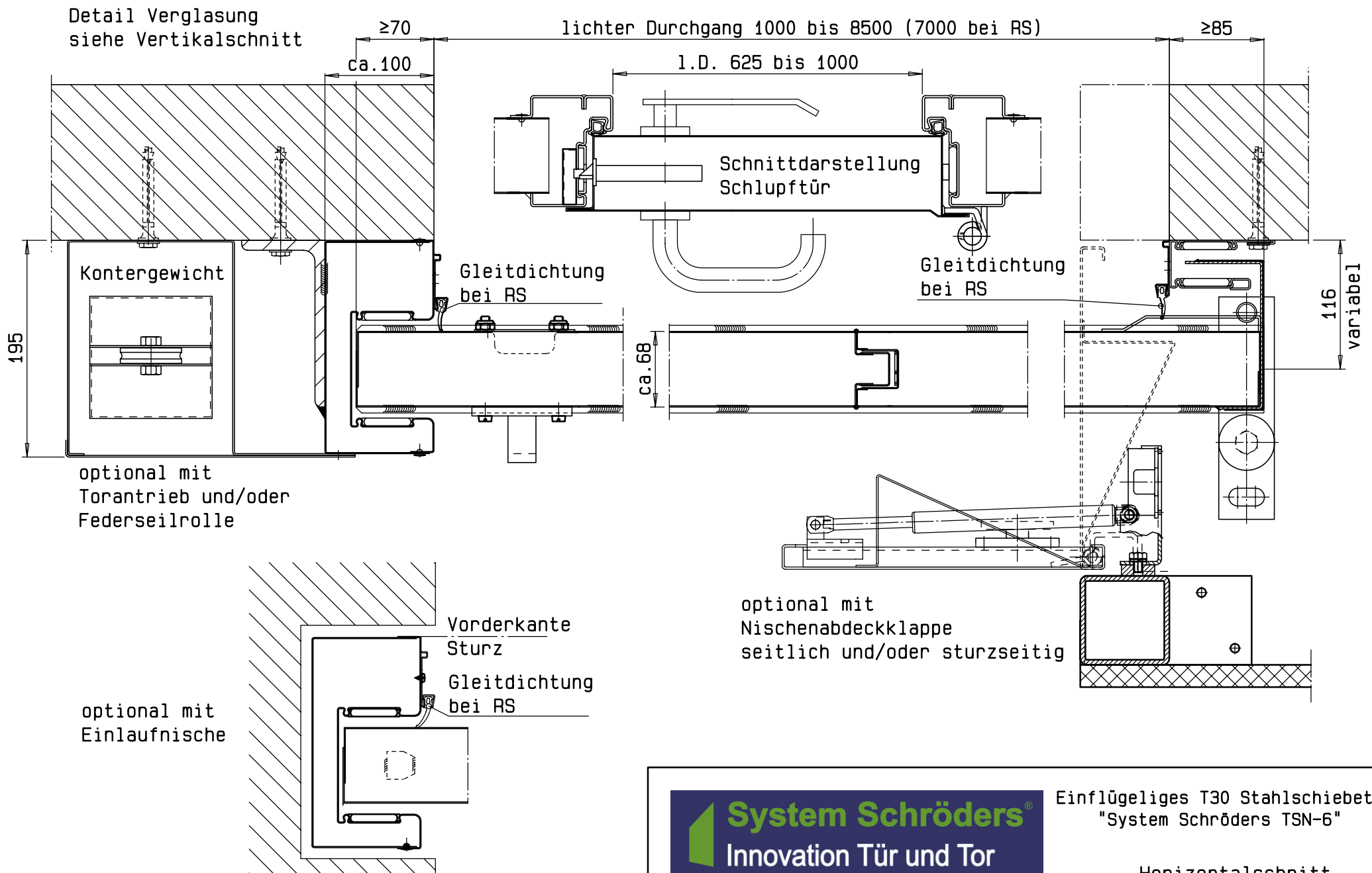
Horizontalschnitt
